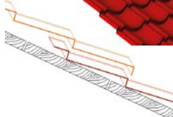
Recouvrement sur 1 tuile
