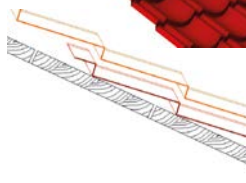
Recouvrement sur 2 tuiles et plus
